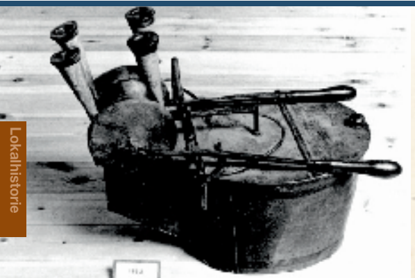
Echardts malkemaskine. Echardt så malkemaskinen på verdensudstillingen i London i 1861 og bestilte en maskine. Den blev senere kopieret, så der var to kopier på Landmandsforsamlingen i Odense i 1863.
